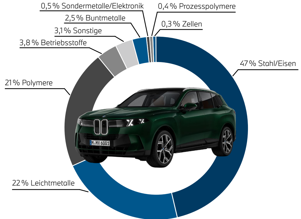
Abb. 2: Werkstoffzusammensetzung des BMW X5 40d xDrive zum Produktionsstart. Die angegebenen Werte können Rundungsdifferenzen aufweisen.
